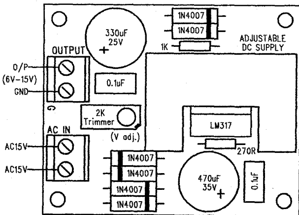
裝配圖
